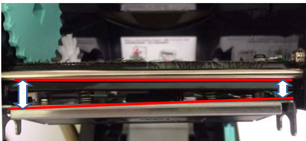
プリンタとブラケットが平行でない 原因)左右どちらかのフックが正しくはまっていない。
